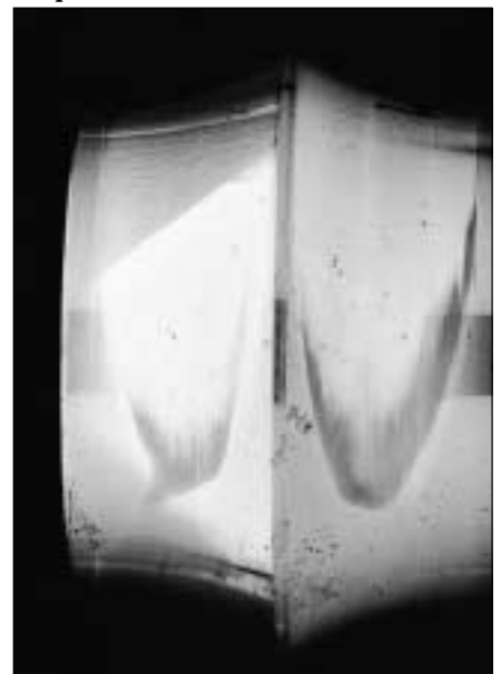
29: Huella de rodadura pulida por la presión
