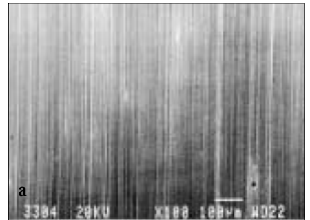
112: Fotografías de estructura superficial obtenidas con el SEM a diferentes aumentos. a: camino de rodadura intacto; b: impresiones de cuerpos extraños duros c: Daños por fatiga en su fase inicial
