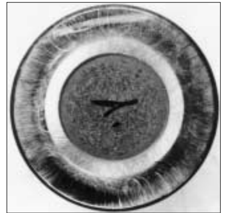
80: Rayas en la superficie frontal de un rodillo cónico
