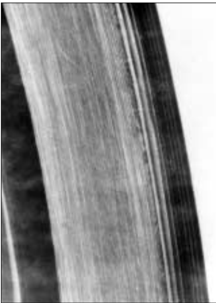
78: Huella de contacto normal en un rodamiento de rodillos cónicos
