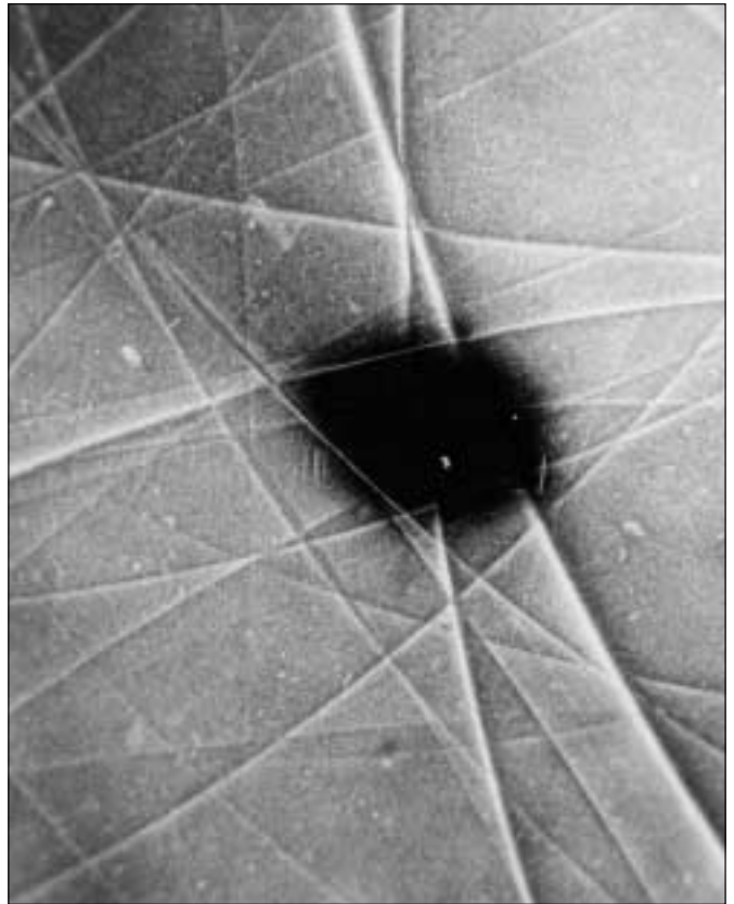
62: Bola con “ovillos completos” de entalladuras, originados por carga variable durante tiempo prolongado
