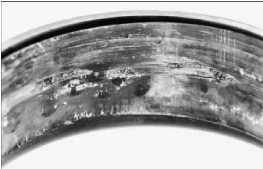
16: Huellas de gripado en el agujero del aro interior como consecuencia del giro relativo del aro interior sobre el eje
