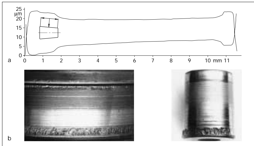
51: El desgaste zonal puede modificar la geometría de las partes que intervienen en la rodadura de tal modo que se produzca fatiga a consecuencia de sobrecarga local a: Registro de forma transversal de un rodillo b: Camino de rodadura del aro interior y rodillo afectados de deterioro por fatiga.
