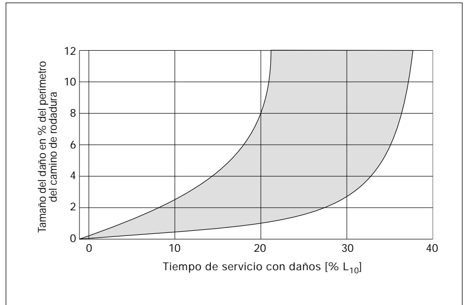
10: Tiempo promedio de servicio remanente de los rodamientos de bolas de contacto angular tras el reconocimiento de un daño por fatiga, en función de la sollicitación, hasta que está dañado 1/10 del perímetro del camino de rodadura. Condición de servicio antes del inicio del primer daño por fatiga: limpieza máxima en el intersticio de lubricación EHD.
