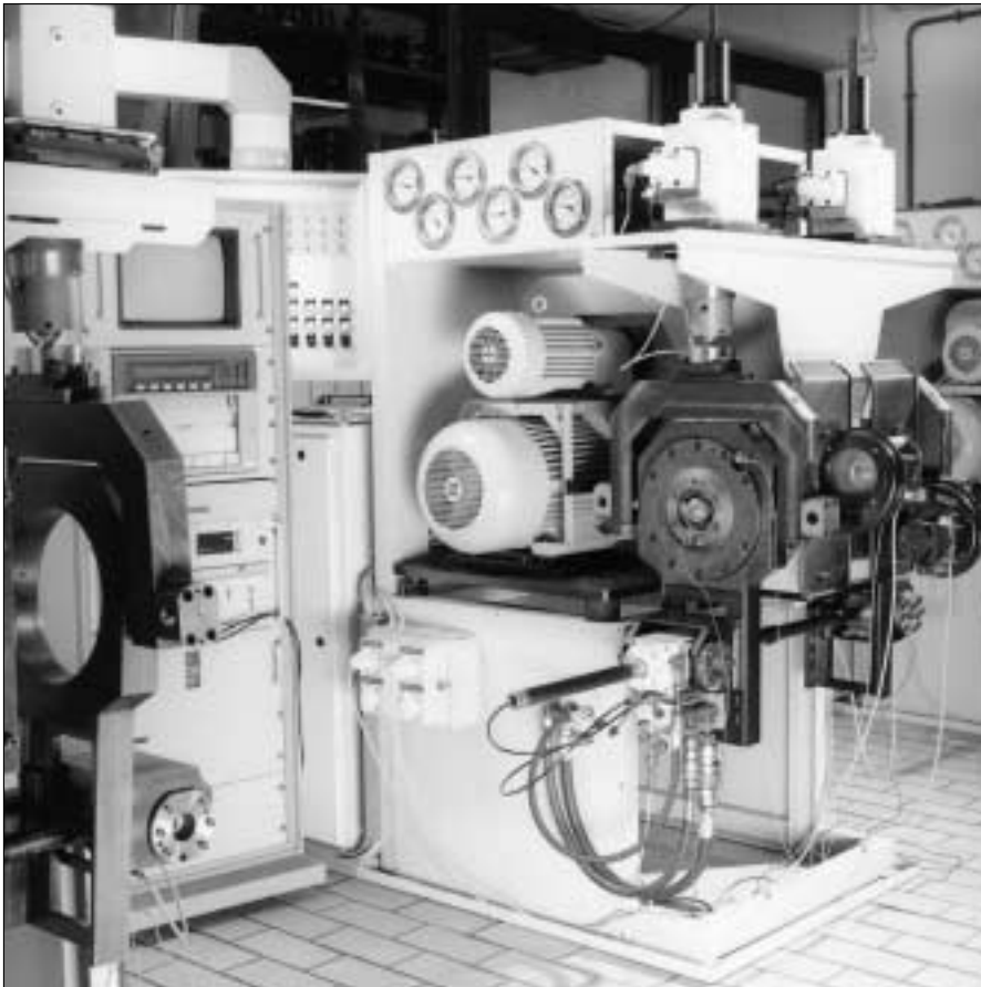
115: Banco de pruebas para la simulación de las sollicitaciones de servicio en rodamientos de ruedas de automóviles
